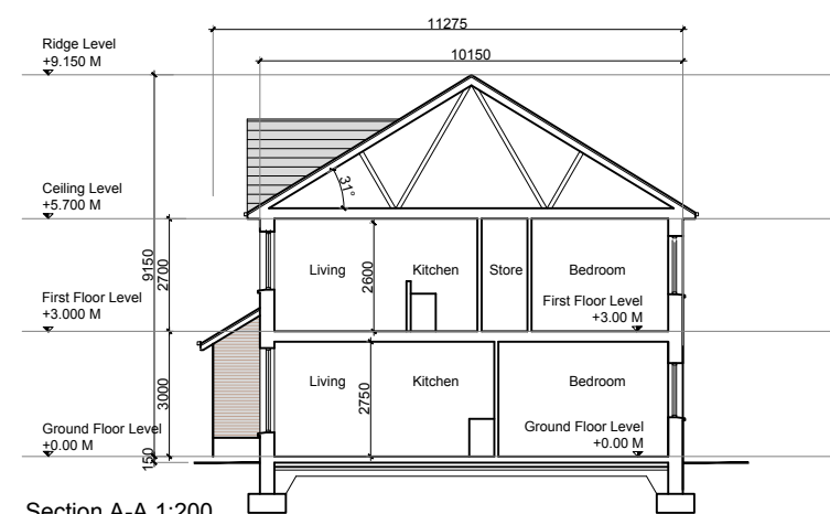
Section A-A 1:200
